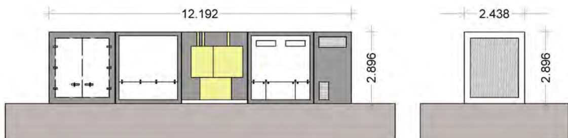
Frontansicht
